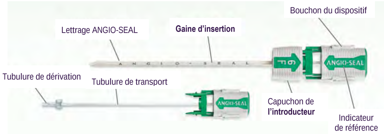
Schéma 1.2 Angio-Seal™ VIP VCD
